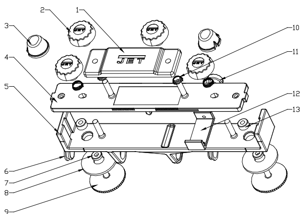
РСJ-1 Приспособление для заточки строгальных ножей
